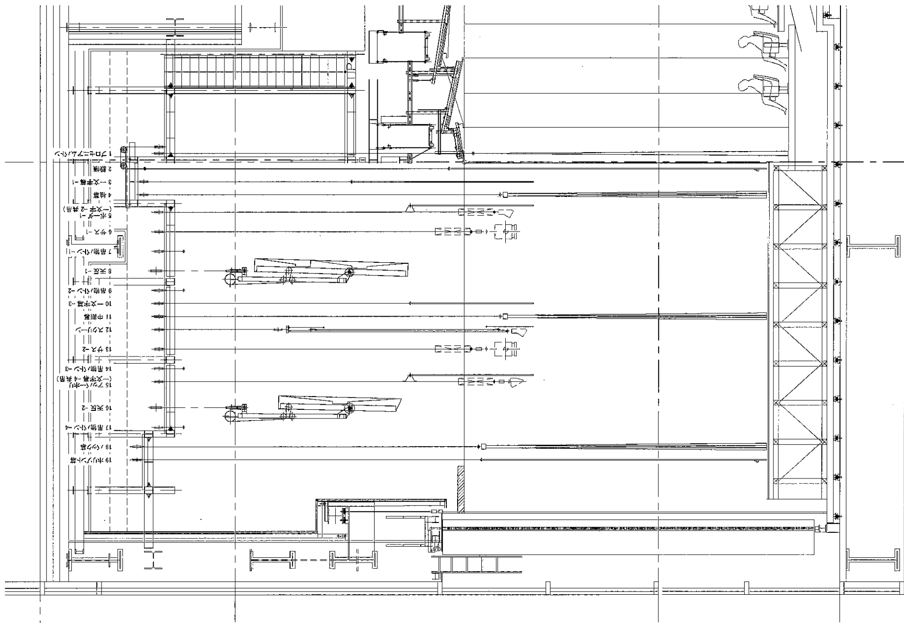
シビックセンターホール 舞台断面図 S=1:60 (A3)
